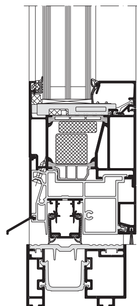
AWS 75.SI+ mit Nullschwelle, Maßstab 1:4 AWS 75.SI+ with zero-level threshold, Scale 1:4
