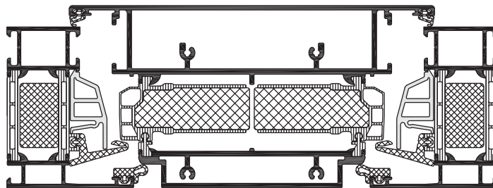
Horizontalschnitt Schüco Lüftungsflügel AWS VV Horizontal section detail of Schüco Ventilation Vents VV
