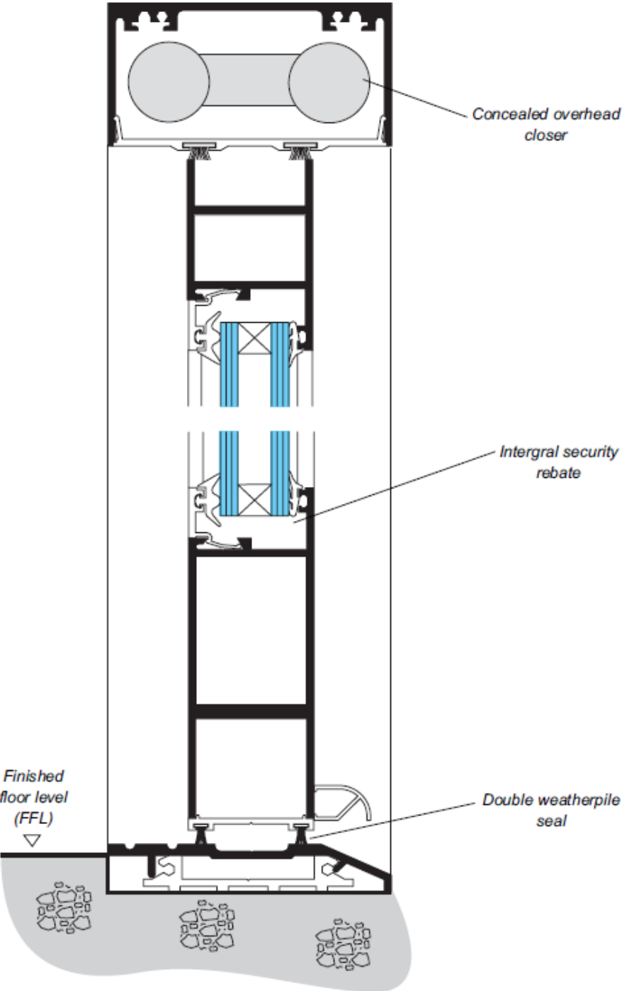
pivot doors. (Scale 1:2)
