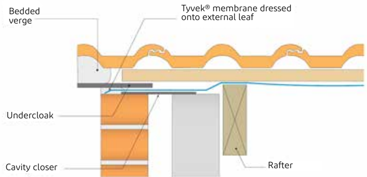
Fig. 42 - Verge
