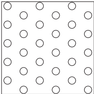
D2016 Ø 2 mm ⇕ 5 ⇔ 8.66 Openness 16%
