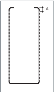
D1522, plain bottom A = 10 mm
