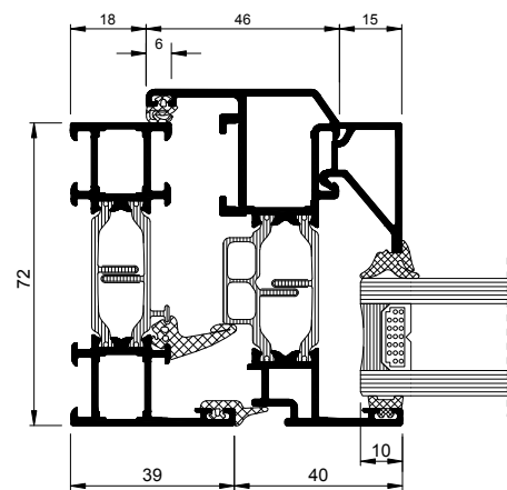
JAMB DETAIL (TILTURN)
