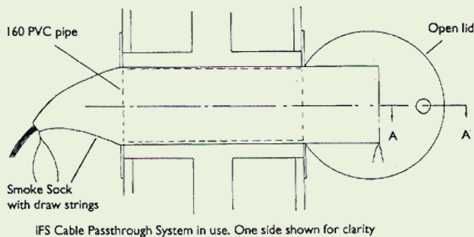
CPTFRW & CPTW DETAIL
