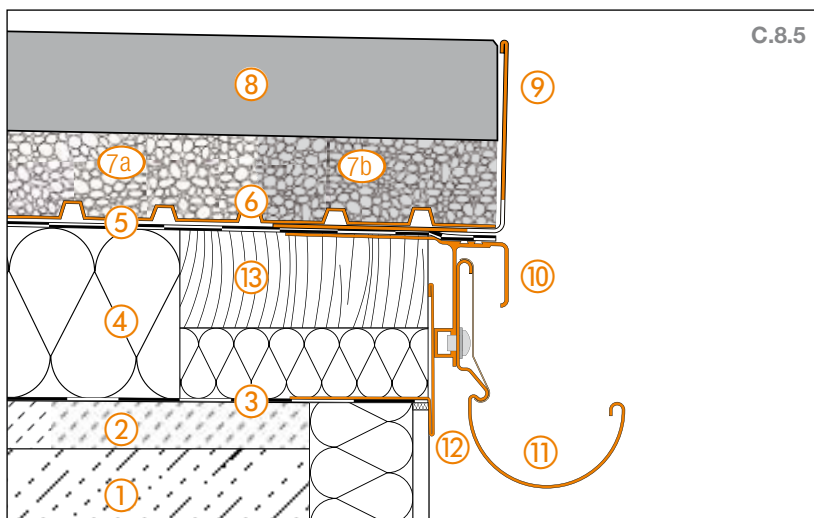
Edge detail 4
