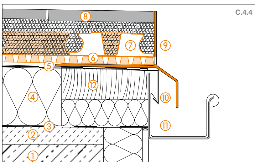
Edge detail 3
