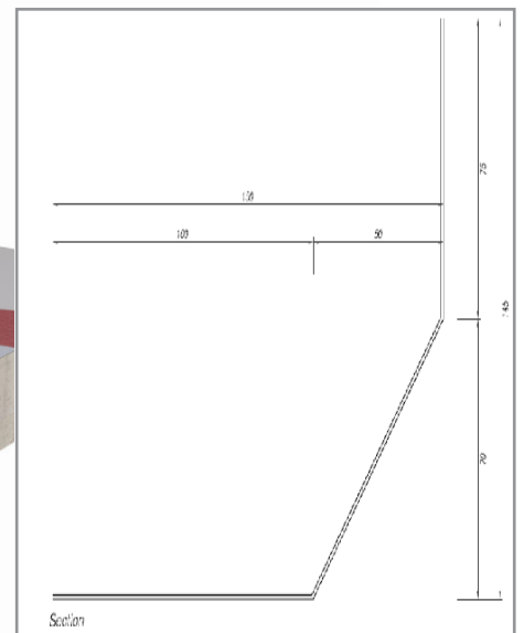
Tortrim UF - Upstand Fillet 75mm
