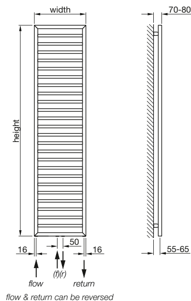
SUB-180 SUBC-180
