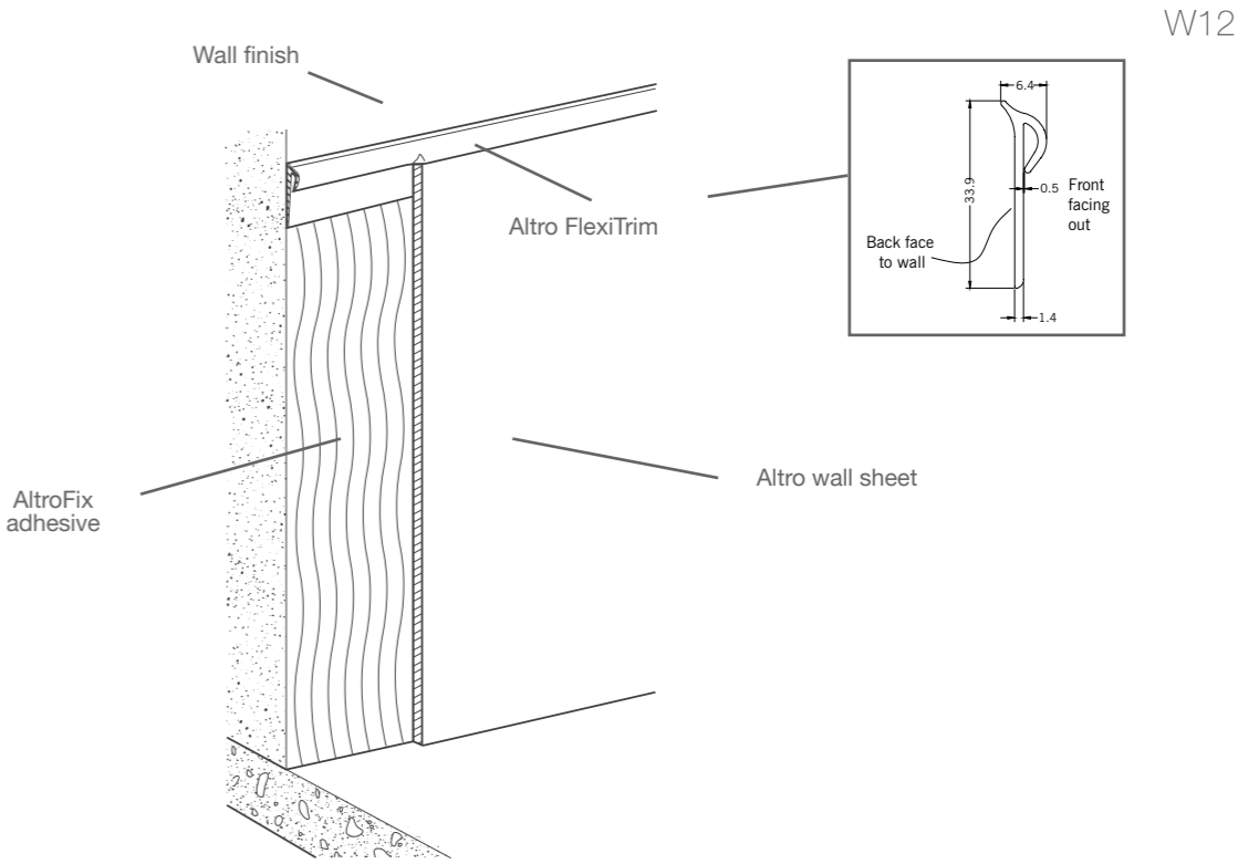
Altro wall sheet at dado height with Altro FlexiTrim
