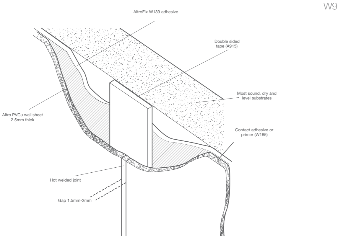
Altro wall sheet to Altro wall sheet detail
